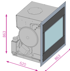
Apertura su parete mm 800 X 810 (LXH)
