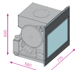
Apertura su parete mm 780 X 700 (LXH)
