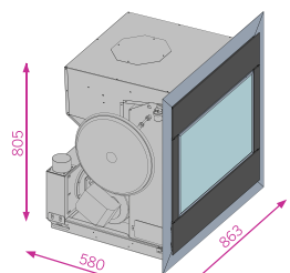
Apertura su parete mm 780 X 700 (LXH)
