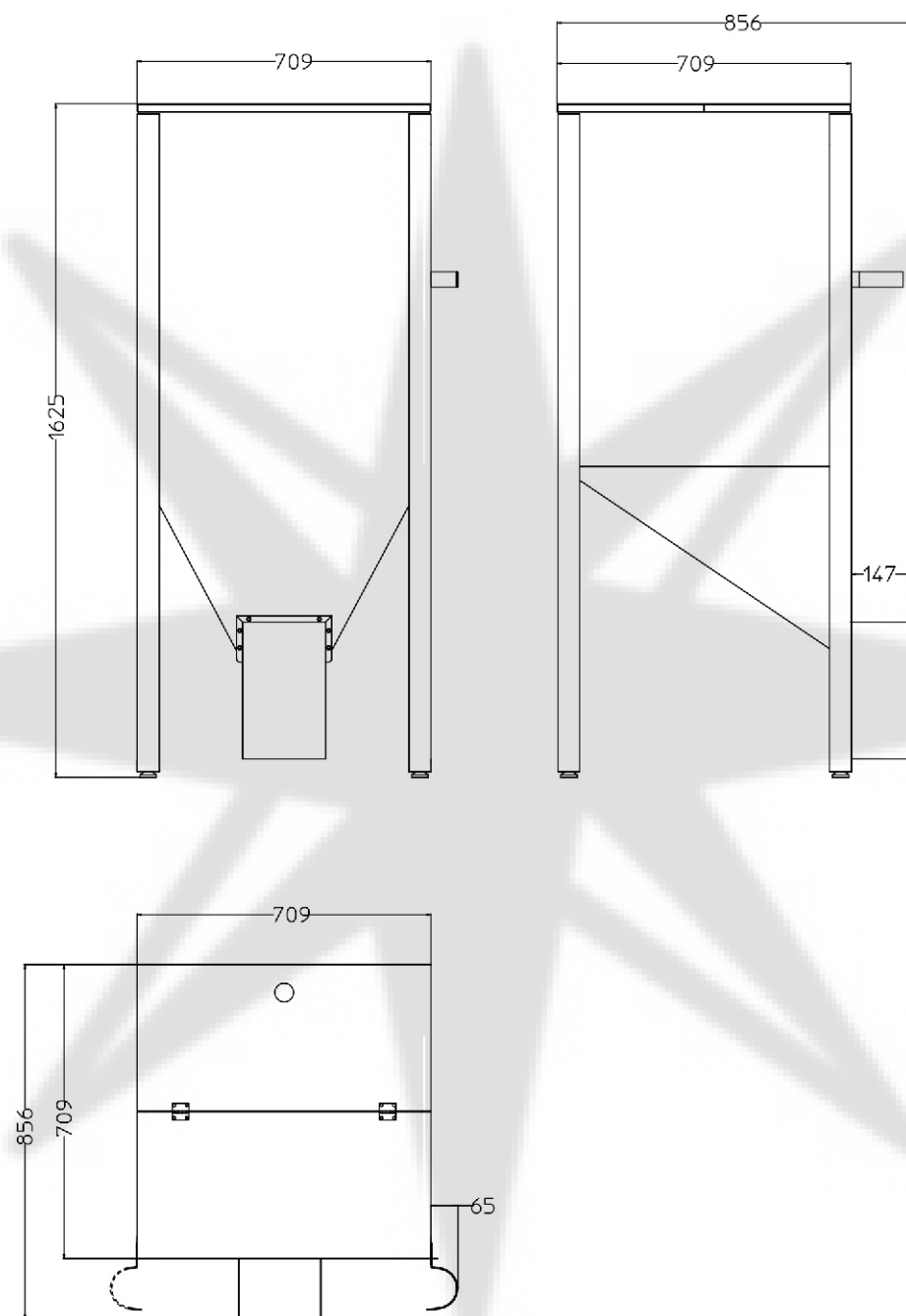
Schema serbatoio 300 kg rev. 09/2010
